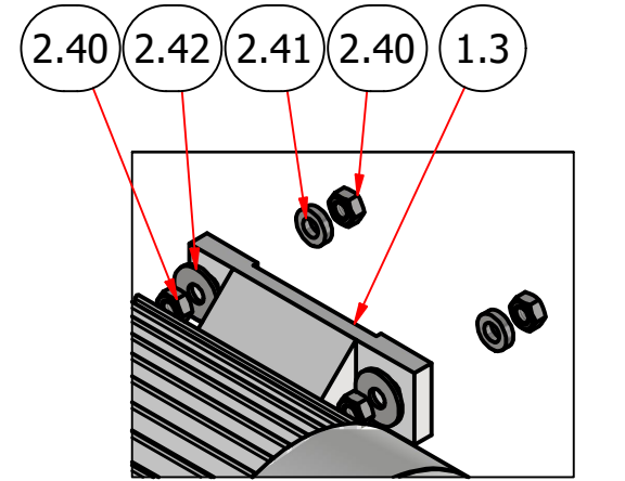
D Detayı (Ölçek 1 : 4 )
